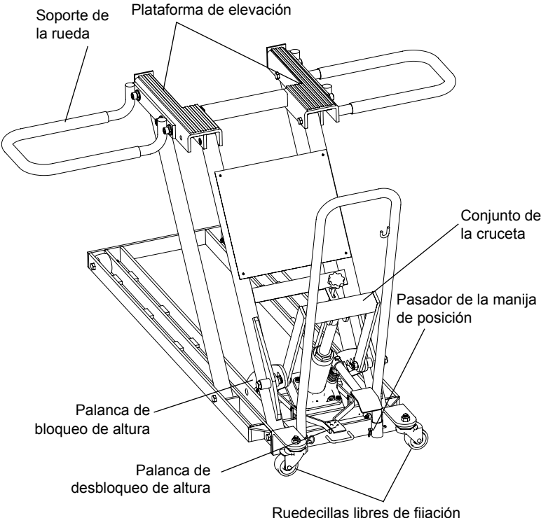
Unidad hidráulica operada por aire Figura 1: nomenclatura de los modelos T-5750
