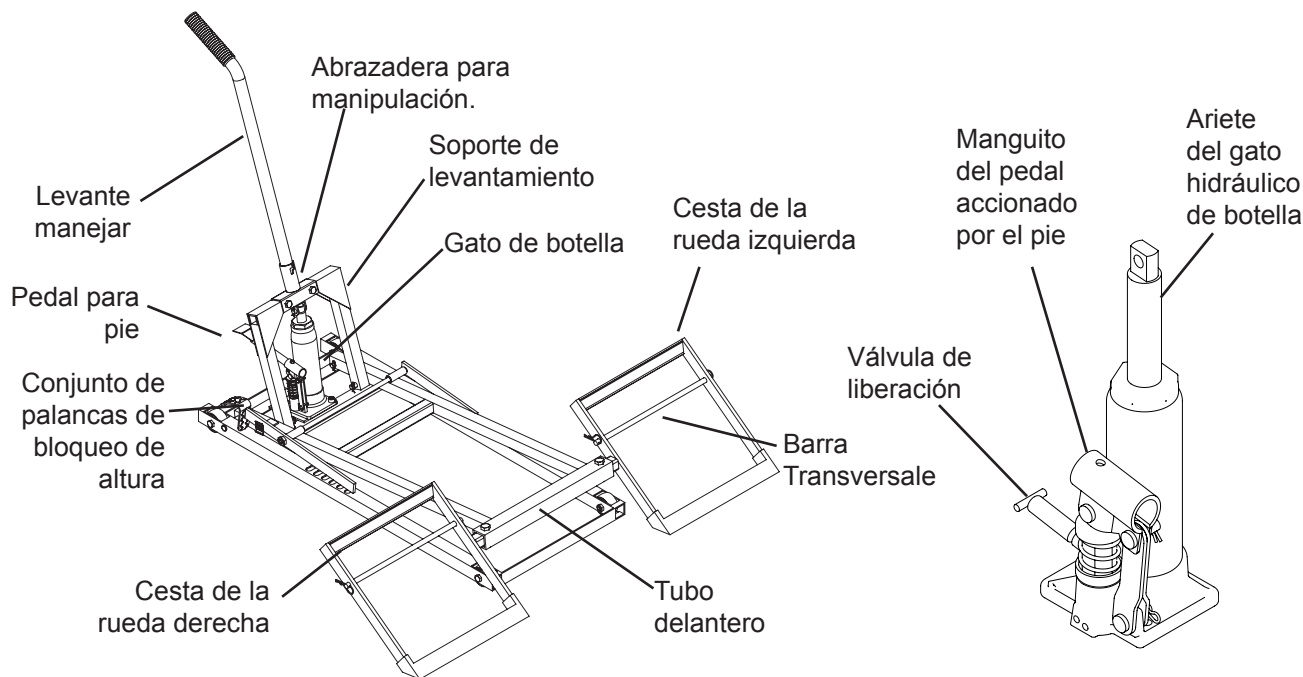
Figura 1: Nomenclatura del elevador del cortacésped.
