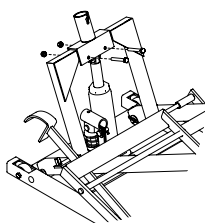
Figura 6: ensamblaje de abrazadera para manipulación.
