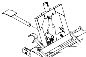
Figura 7: ensamblaje del pedal accionado por el pie.
