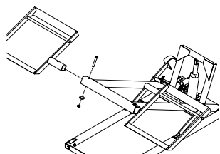
Figura 5: colocación de la abrazadera para ruedas
