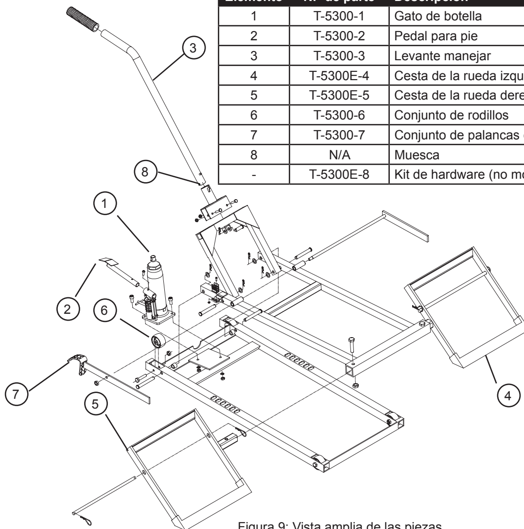
Figura 9: Vista amplia de las piezas.
