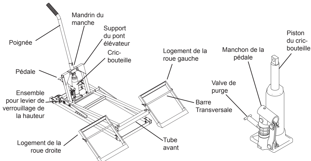
Figure 1 : Nomenclature du pont élévateur à tondeuse
