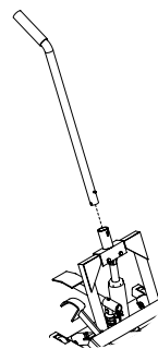
Figura 8: ensamblaje de la manija.
