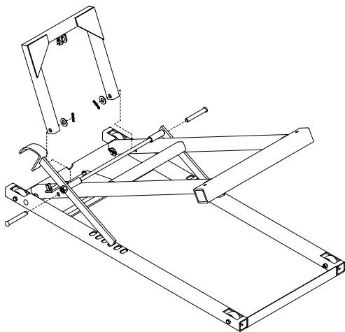
Figura 2: ensamblaje del soporte de levantamiento.
