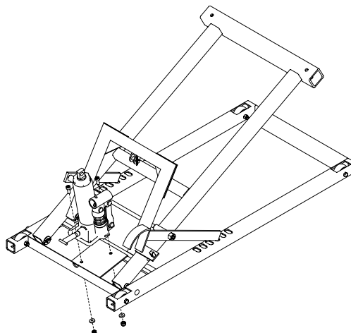
Figure 3 : Assemblage du cric-bouteille à la plate-forme
