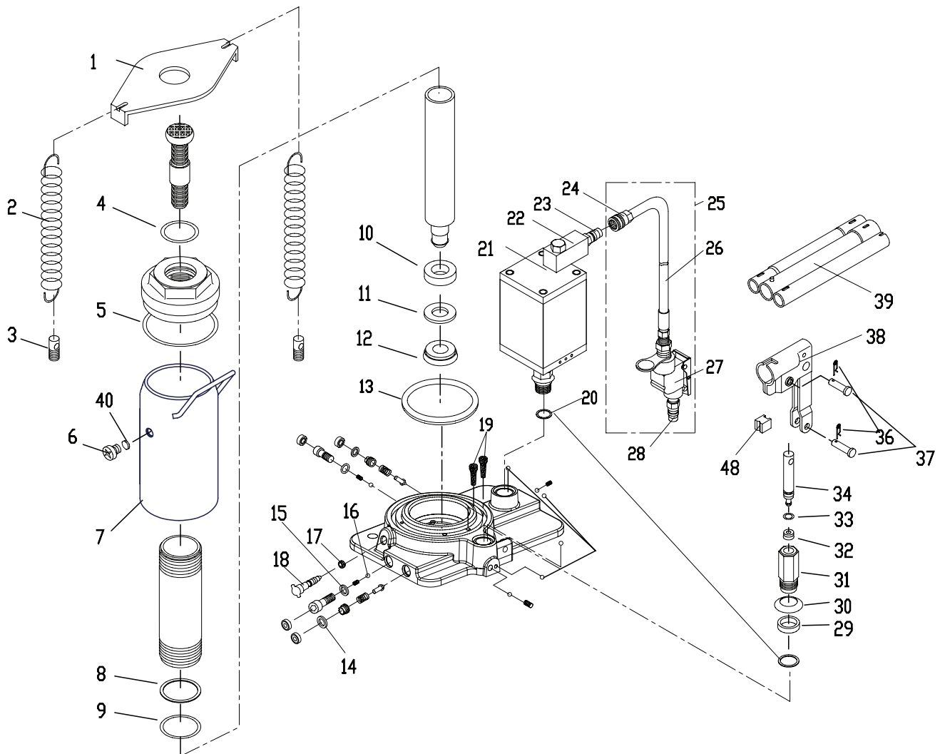
Figure 2 - Illustration des pièces de rechange
