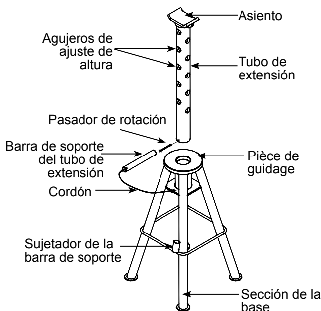
Figure 1 : Composantes de los modelos 32105B y 32107B
