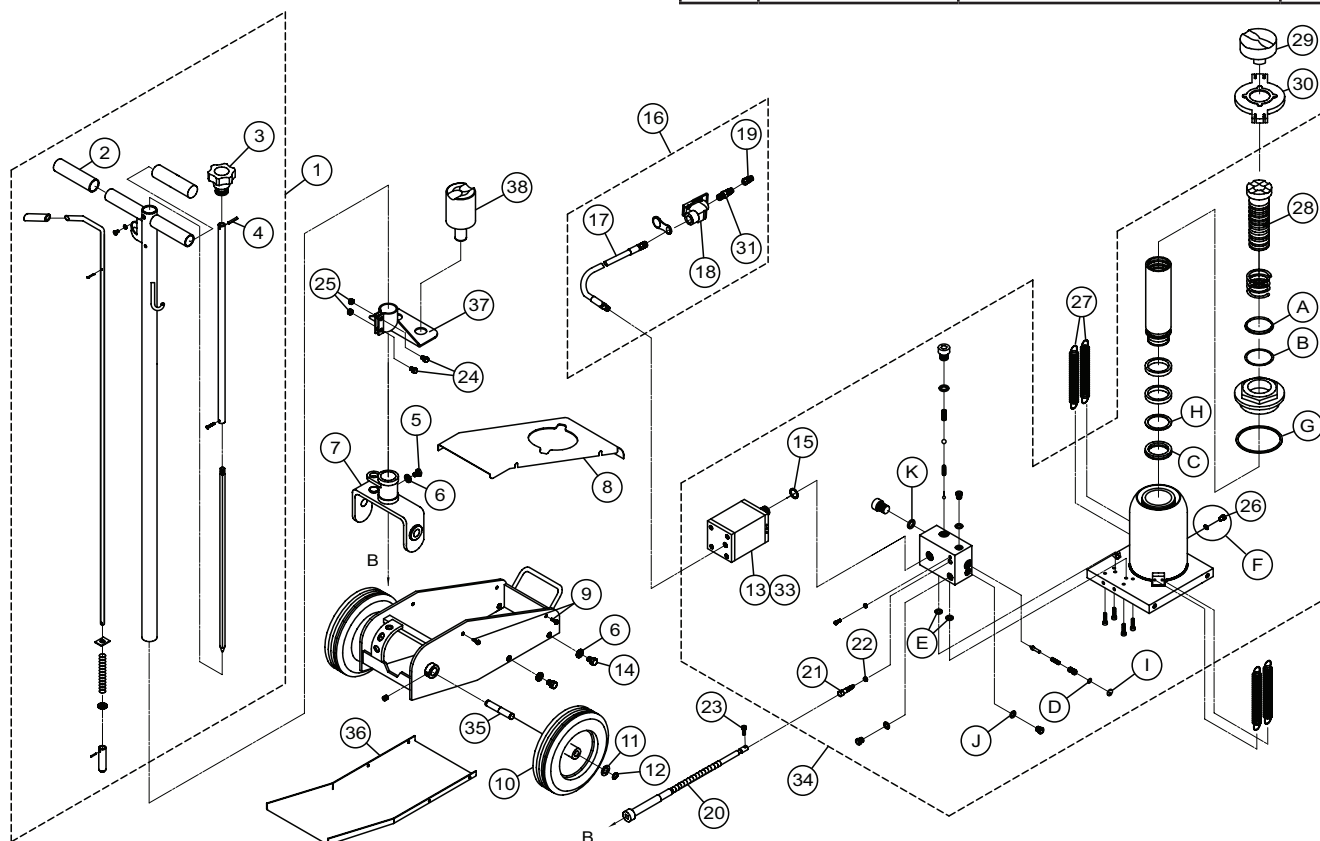
Figure 2 : Illustration des pièces de rechange des modèles 23221C et 23222C
