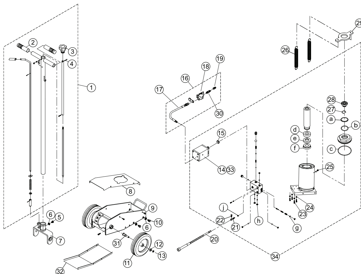
Figure 3 : Illustration des pièces de rechange du modèle 23301C
