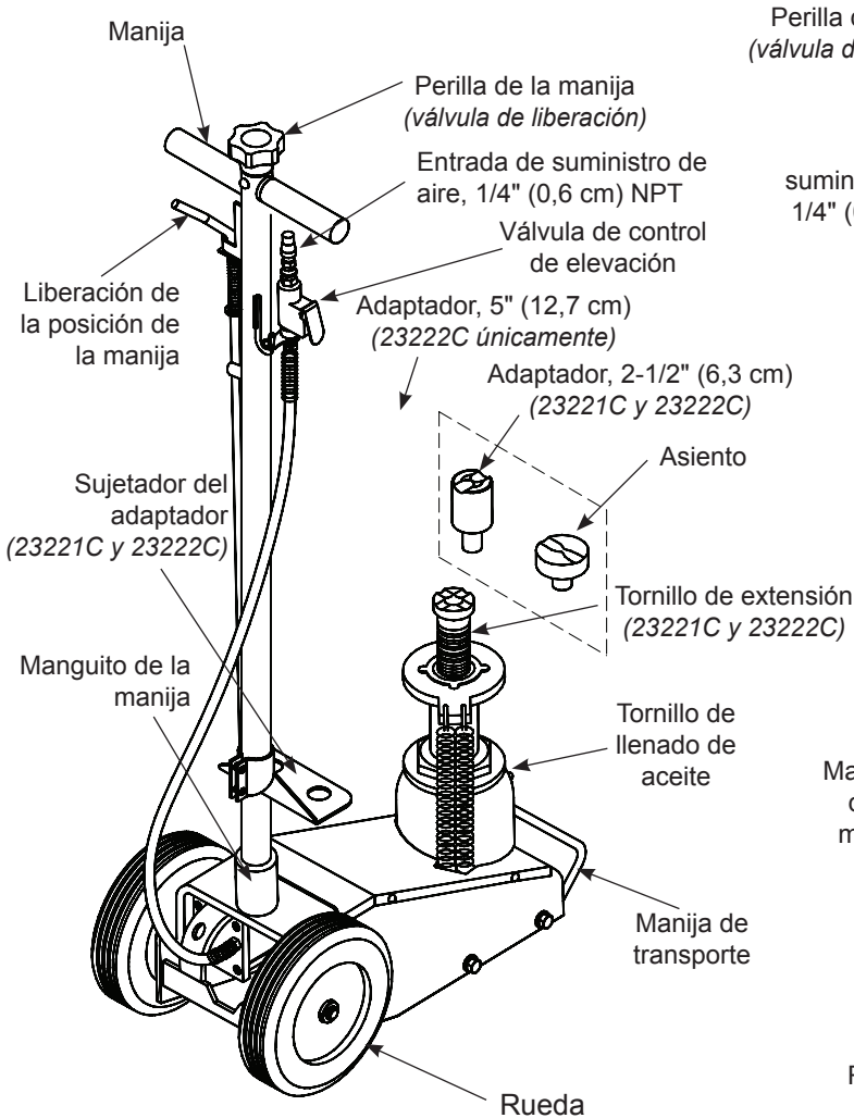
Figura 1: Nomenclatura habitual de un gato para camiones (se muestra 23222C)
