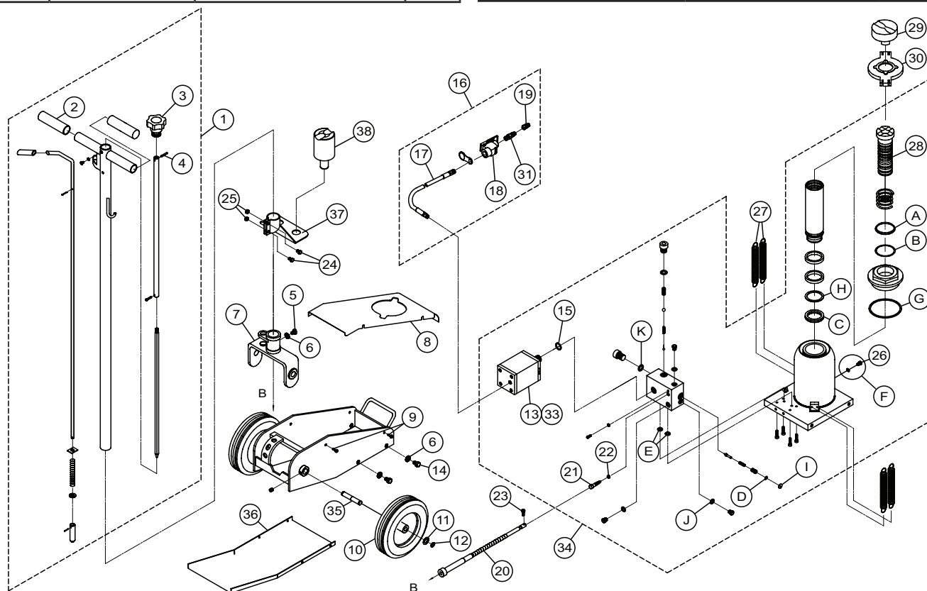
Figura 2: Ilustración de piezas de repuesto para los modelos 23221C y 23222C
