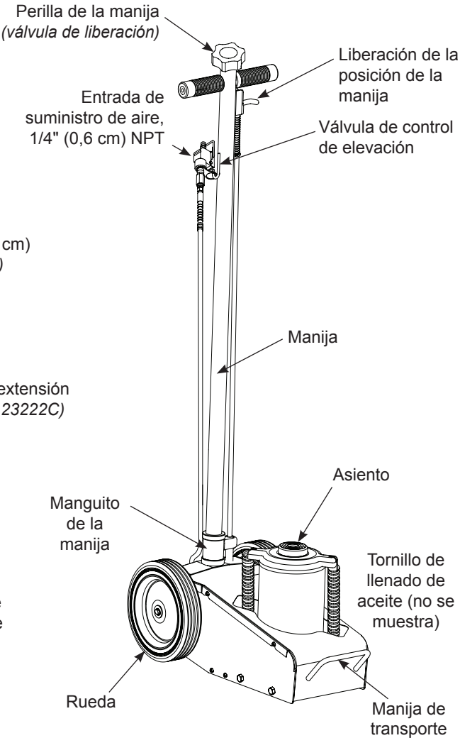
Figura 1: Nomenclatura del modelo 23301C
