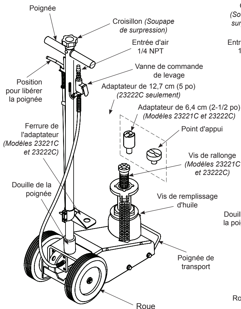
Figure 1 : Pièces d'un cric hydraulique pour camion typiques (modèle 23222C)
