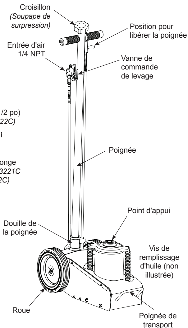
Figure 1 : Pièces d'un cric hydraulique pour camion typiques (modèle 23301C)
