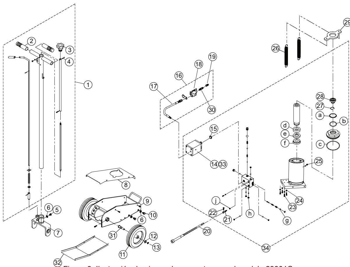
Figura 3: Ilustración de piezas de repuesto para el modelo 23301C
